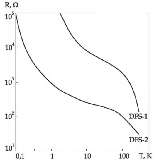
Температурна залежність опору для двох типів багатифункціональних сенсорів моделі DFS-1 і DFS-2
