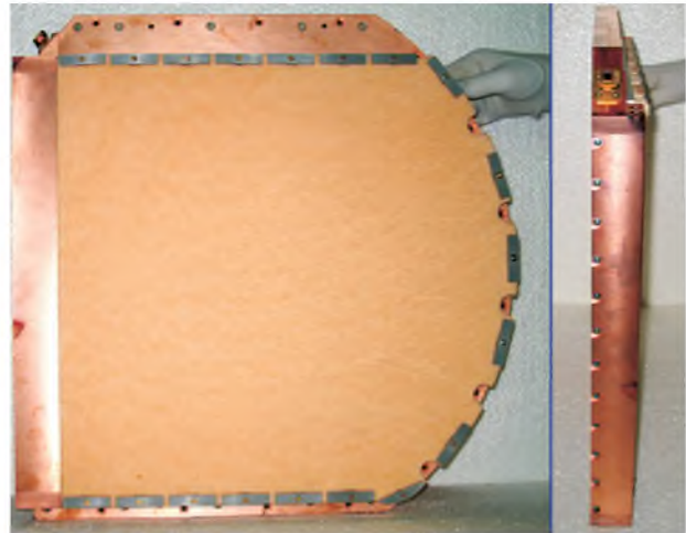
Дифракційна антена W-діапазону для багатопроменевих пасивних систем візуалізації
