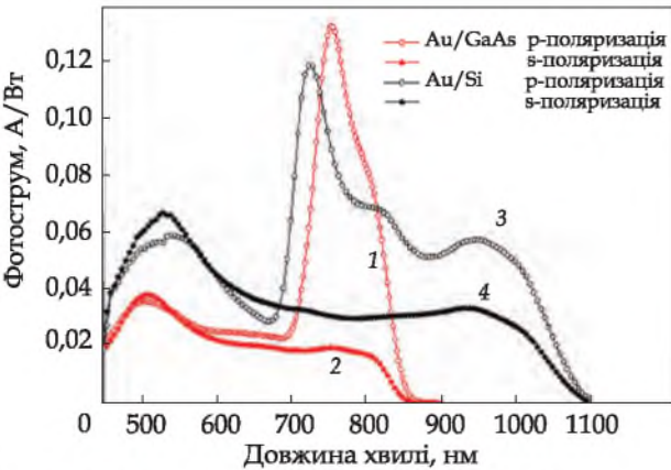
Спектральні характеристики фотоструму ППФ Au/GaAs (1,2) та Au/Si (3,4) для світла р-(1,3) та s-(2,4) поляризації
