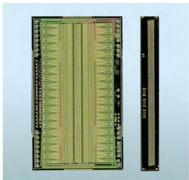
Багатоелементні приймачі ІЧ-випромінювання для спектрального діапазону 3–5 та 8–12 мкм
