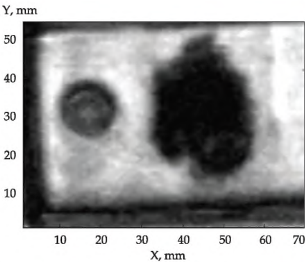
Зображення предметів, розташованих у пінопластовому пакунку, отримані за частоти випромінювання 140 ГГц
