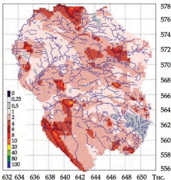
Модель розрахункової області Nadra-3D
