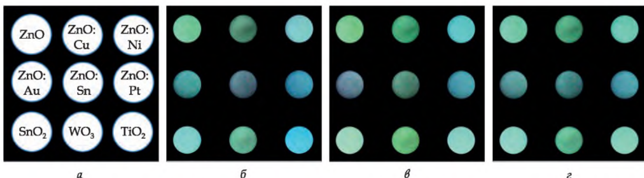
Фотолюмінесцентне свічення комірок сенсорної матриці (а) в газовому середовищі (б – повітря, в – CO, г – вакуум)
