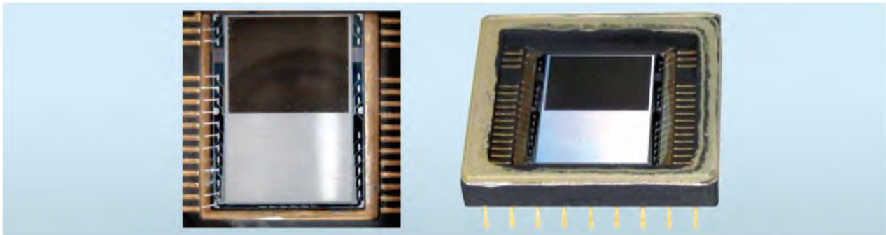
Фотоматриці ПЗЗЕМ (вигляд в корпусі зверху та збоку)
