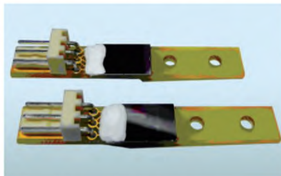
Уніфіковані первинні електроди для приладу
