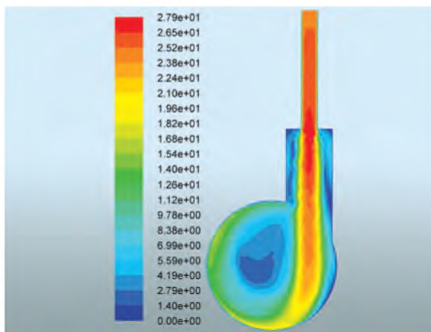
Моделювання горіння метану в реакторі циклонного типу
