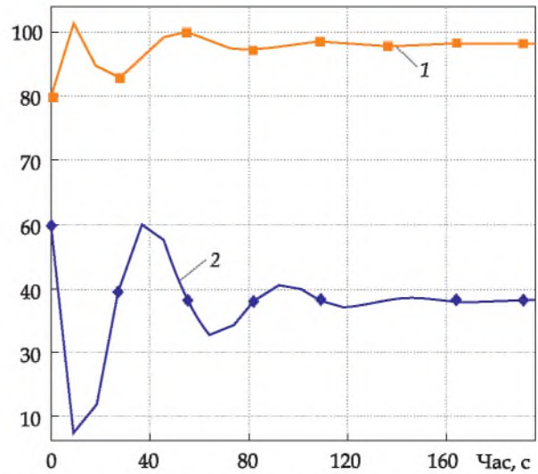
Симуляція моделі гемодинаміки: динаміка середнього артеріального тиску (1) та частоти скорочень серця (2)
