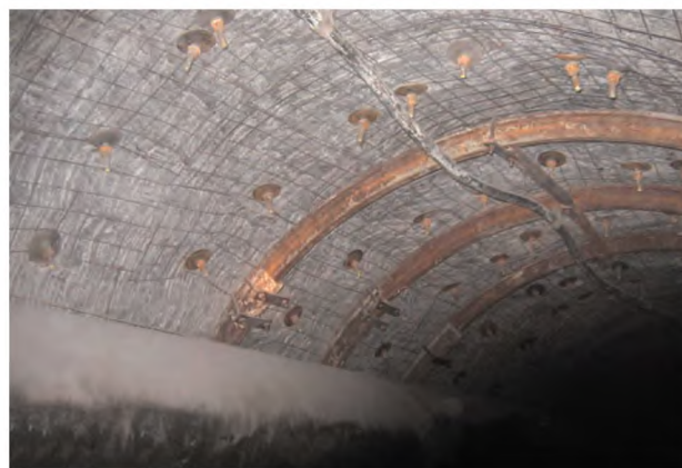
Виробки з анкерним (вгорі) та анкерно-рамним (внизу) кріпленням
