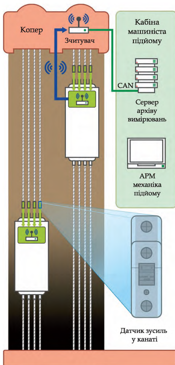
Схема технології безперервного контролю натягів каналів у шахтних багатоканатних підйомних установках
