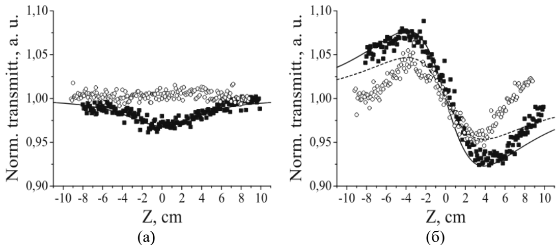
Рис. 10. Нелінійний відгук Ag-нанокомпозиту при збудженні на довжині хвилі 800 нм ( \tau = 180 \text{ фс} , f = 75 \text{ кГц} , I_0 = 0,142 \text{ ГВт/см}^2 ): із відкритою діафрагмою (а) та із закритою діафрагмою (СА/ОА) (б) Результати Z-сканування для хаотичних (незафарбовані кола) і впорядкованих (чорні квадрати) структур. Лінії відповідають теоретичному наближенню.
