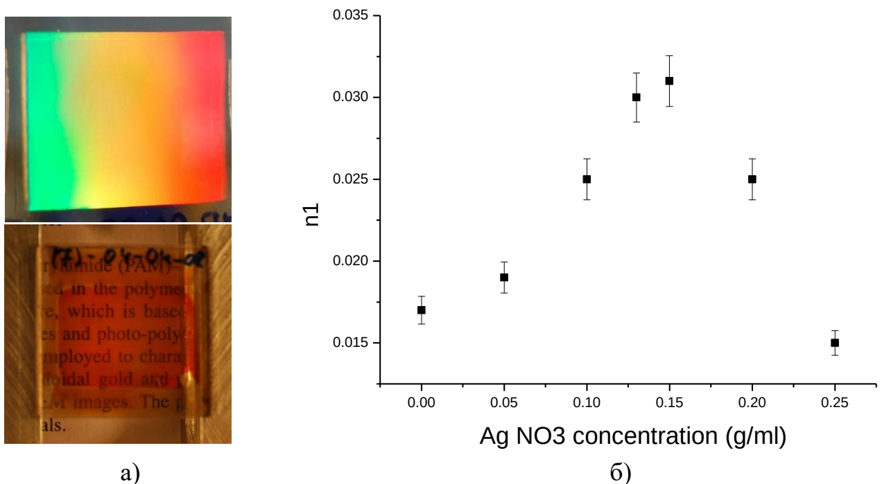
Рис. 4. Фото ґратки, сформованої НЧ Ag в полімерній матриці, її оптична якість (а). Залежність n_1 ґратки від концентрації \text{AgNO}_3 в розчині прекурсору (б).
