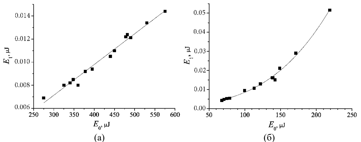
Рис. 8. Нелінійна рефрактометрія полімерних шарів із d = 20 мкм, які містять НЧ Au різного розміру: (а) діаметр НЧ (1,7 \pm 0,3) нм, (б) діаметр НЧ (2,7 \pm 0,8) нм.
