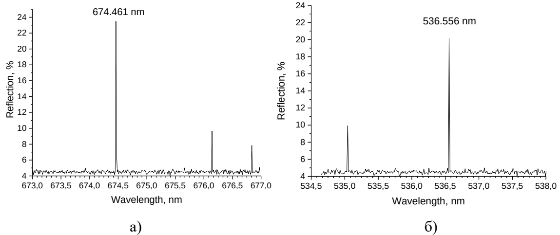
Рис. 11. Довгохвильові (а) і короткохвильові (б) резонансні смуги у спектрі відбиття від РХГ при падінні світлової хвилі під кутом 10^\circ .
