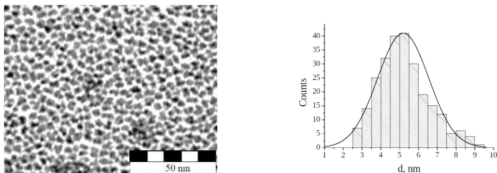
Рис. 1. Електронно-мікроскопічне (ТЕМ) зображення НЧ і гістограма розподілу НЧ за розміром (площа ділянки спостереження 3,5 \text{ мкм} \times 3,5 \text{ мкм} , середній діаметр 5,24 нм, стандартне відхилення 1,37 нм).
