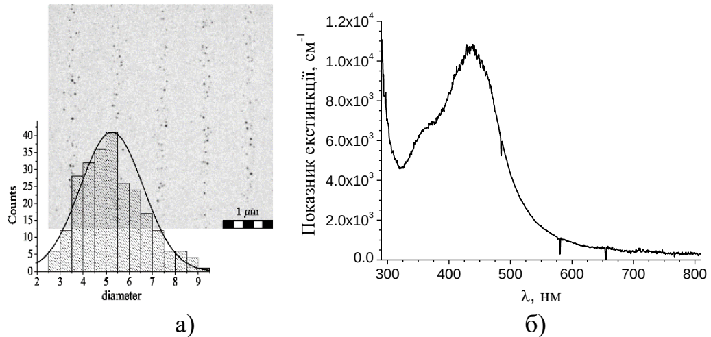
Рис. 3. (а) ТЕМ-зображення ґратки з утвореними in situ НЧ Ag і гістограма розподілу НЧ за розмірами (площа 3,5 мкм \times 3,5 мкм; середній діаметр 5,25 нм; стандартне відхилення становить 1,3 нм); (б) показник екстинкції нанокompозитної плівки, що містить НЧ Ag.
