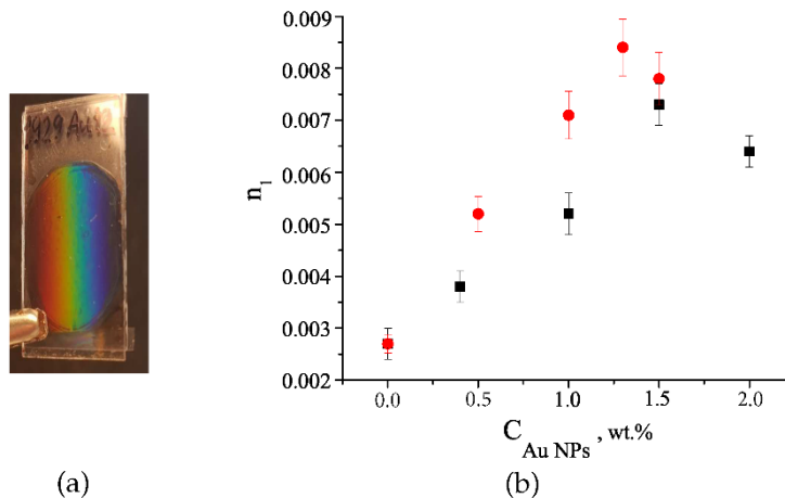
Рис. 2. Фото ґратки у наноккомпозиті з НЧ Au (а). Максимальні значення n_1 як функція концентрації НЧ Au для Au1 (чорні квадрати) та Au2 (червоні круги) (б).
