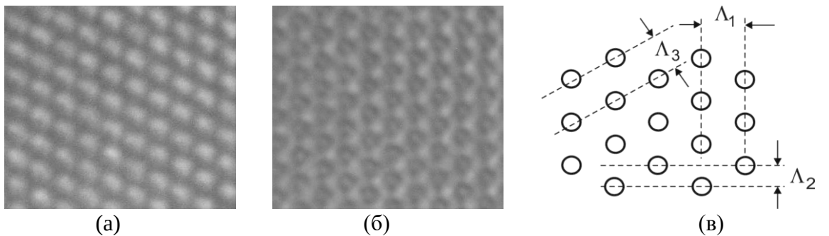
Рис. 6. Мікрофотографії 2D кристалів (атомно силовий мікроскоп), сформованих розподілом НЧ Ag у полімерній матриці: \Psi_{3,0} (а), \Psi_{6,3} (б); кристалічна ґратка для \Psi_{3,0} (в).
