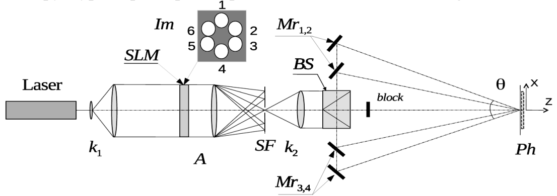
Рис. 5. Схема багатопучкового голографічного запису 2D структур: Laser — Ar+ лазер, k_1 , k_2 — коліматори, SLM — просторовий модулятор світла, із заданим просторовим розподілом фаз Im , SF — просторовий фільтр, BS — призмова система розділення лазерного пучка, Mr_{1-6} — дзеркала, \theta — кут між пучками та віссю Z, Ph — фоточутливе середовище.
