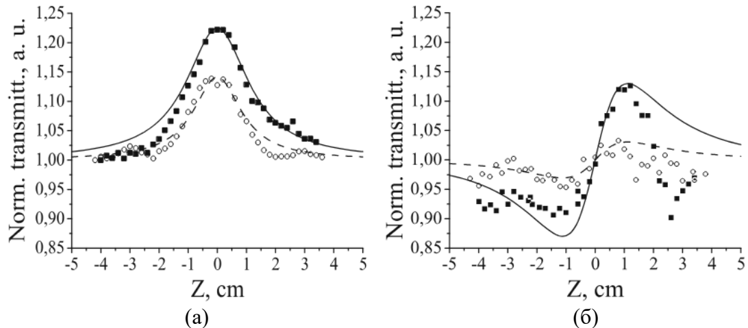
Рис. 9. Нелінійний відгук Ag-нанокомпозиту при збудженні на довжині хвилі 532 нм ( \tau = 20 \text{ нс} , f = 0,5 \text{ Гц} , I_0 = 5,11 \text{ МВт/см}^2 ): із відкритою діафрагмою (а) та із закритою діафрагмою (СА/ОА) (б). Результати Z-сканування для хаотичних (незафарбовані кола) і впорядкованих (чорні квадрати) структур. Лінії відповідають теоретичному наближенню.
