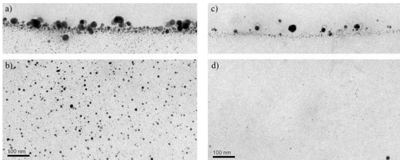
Рис. 7. ТЕМ зображення структури полімерної плівки. (а), (б) – Біля передньої підкладки, зверненої до освітлення. (с), (д) – У центрі шару. (а), (с) – Інтенсивність лазерного випромінювання становить 7 мВт/см 2 . (б), (д) – Інтенсивність лазерного випромінювання становить 14 мВт/см 2 .
