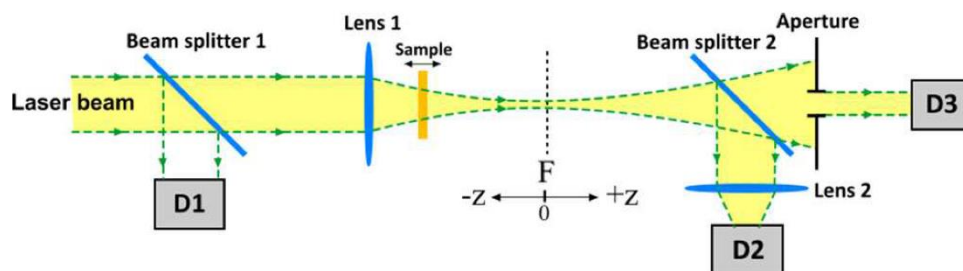
Рис. 2.2. Схема методу Z-сканування: D1, D2, D3 – детектори. [102]
