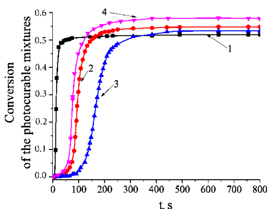
Рис. 3.6. Перетворення: суміші мономерів (1); нанокompозиту з 1,5 мас.% Au1 (2) і 2 мас.% Au1 (3); нанокompозиту з 1,3 мас.% Au2 (4).
