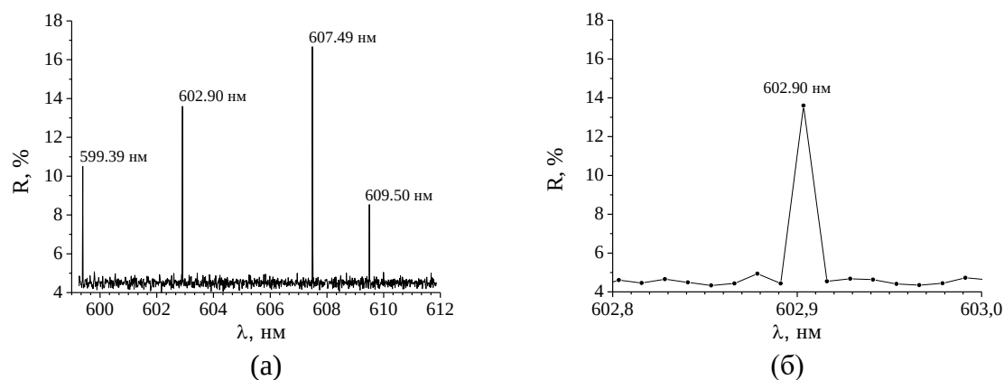
Рис. 5.14. Спектр відбиття отриманий для кута падіння 0,25^\circ (а); ділянка спектру поблизу короткохвильової смуги (б).
