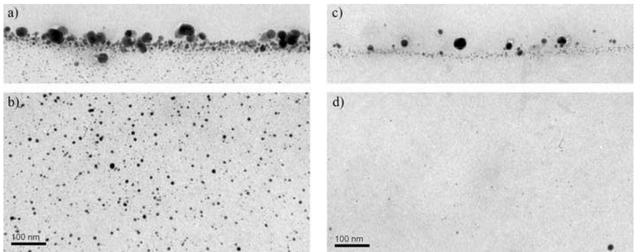
Рис. 3.15. ТЕМ зображення структури полімерної плівки. (а), (б) – Біля передньої підкладки, зверненої до освітлення. (с), (d) – У центрі шару. (а), (с) – Інтенсивність лазерного випромінювання становить 7 мВт/см 2 . (b), (d) – Інтенсивність лазерного випромінювання становить 14 мВт/см 2 .
