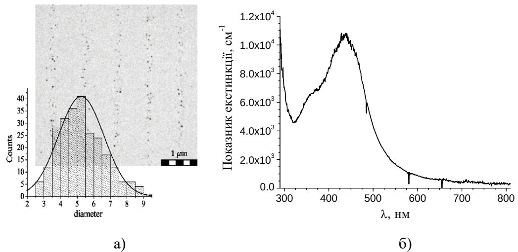
Рис. 3.10. (а) ТЕМ-зображення ґратки з утвореними in situ НЧ Ag і гістограма розподілу НЧ за розмірами (площа 3,5 мкм × 3,5 мкм; середній діаметр 5,25 нм; стандартне відхилення становить 1,3 нм); (б) показник екстинкції нанокompозитної плівки, що містить НЧ Ag.
