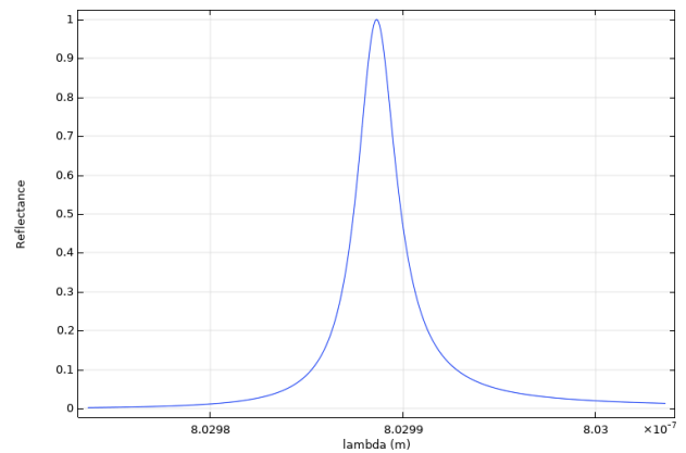
Рис.5.10. Спектральна залежність коефіцієнта відбиття при куті падіння пучка на ґратку в досліджуваному середовищі 20,171^\circ , що відповідає куту в повітрі 30^\circ . Півширина спектра складає 0,0025 нм.
