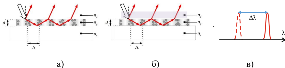
Рис. 5.1. Схематичне зображення РХГ без (а) та із досліджуваною речовиною на її поверхні (б): d – товщина шару; \Lambda – період структури; n_a , n_g та n_s – показники заломлення зовнішнього середовища, ґратки та підкладки, відповідно. Спектральний зсув резонансної смуги при зміні показника заломлення зовнішнього середовища n_a (в).
