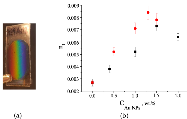
Рис. 3.4. Фото ґратки у нанокompозиті з НЧ Au (a). Максимальні значення n_1 як функція концентрації НЧ Au для Au1 (чорні квадрати) та Au2 (червоні круги) (b). [102]
