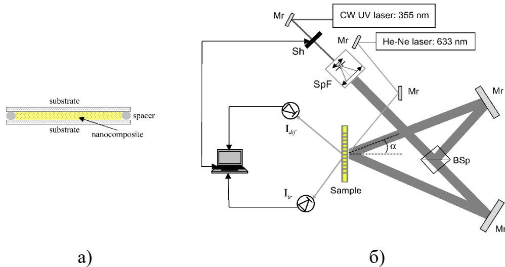
Рис. 2.1. а) Поперечний переріз фоточутливого шару. б) Оптична схема установки голографічної літографії для запису 1D періодичних структур: SpF — просторовий фільтр і блок телескопа, Mr — дзеркала, BSp — світлоподільний кубик, що розділяє вхідний лазерний промінь на два однакових за інтенсивністю пучка, sample — шар, що реєструє інтерференційну картину, He-Ne лазер для зчитування ґратки в процесі експонування. [102]
