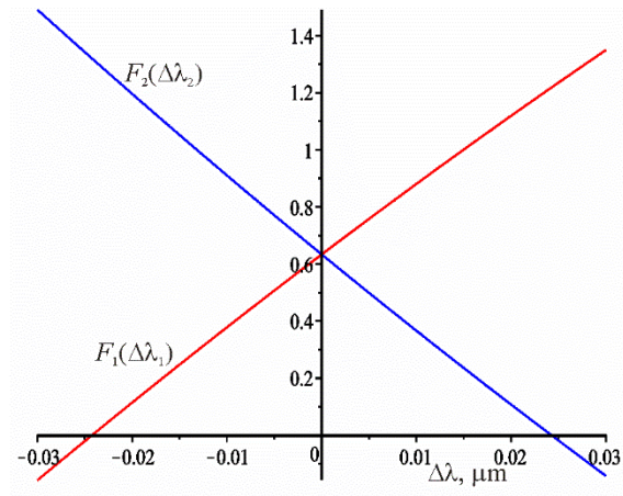
Рис. 5.2. Графічні залежності F_1(\Delta\lambda_1) і F_2(\Delta\lambda_2) , кут падіння на хвильовод у повітрі складає 3,5^\circ .
