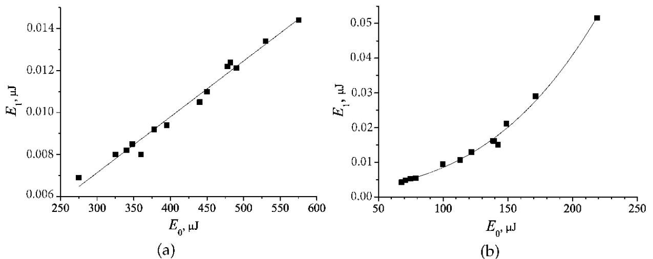
Рис. 4.1. Нелінійна рефрактометрія полімерних шарів із d = 20 мкм, які містять НЧ Au різного розміру: (а) діаметр НЧ (1,7 \pm 0,3) нм, (б) діаметр НЧ (2,7 \pm 0,8) нм.
