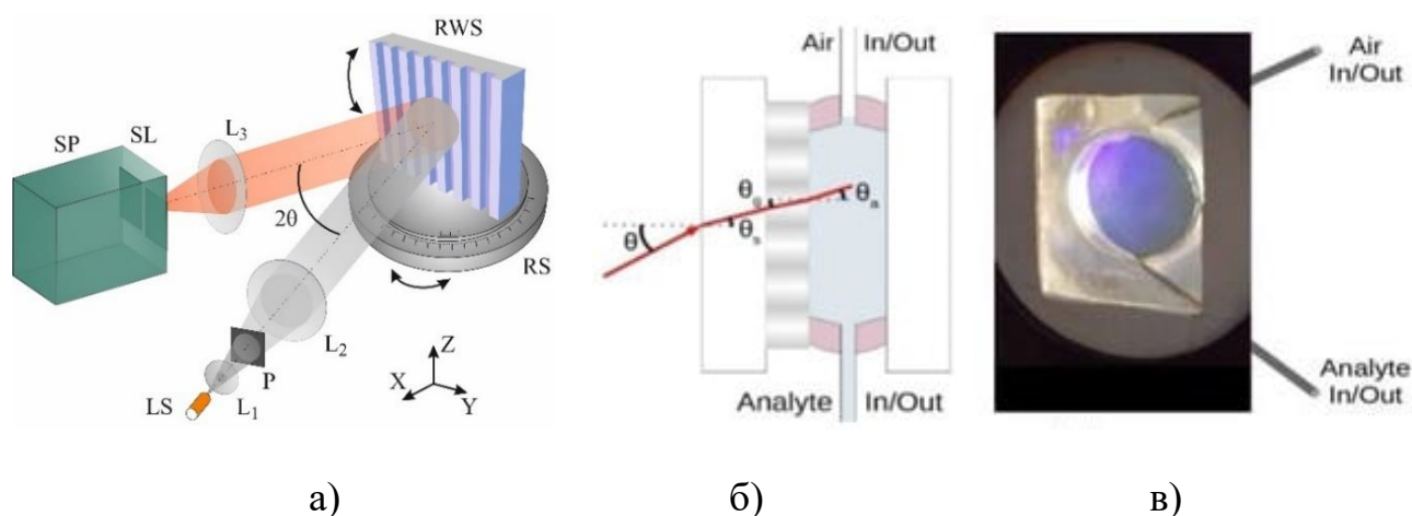
Рис. 2.3. Схема спектральної установки для вимірювання спектрів відбиття (а) і вимірювальна кювета у поперечному розрізі (б) та вигляд у зборі зі сторони PXI (в).
