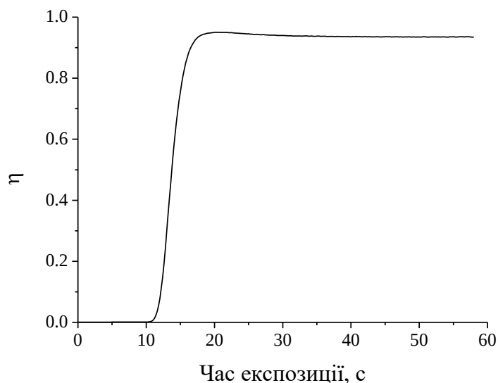
Рис.3.8. Типова крива кінетики дифракційної ефективності при записі ґраток із НЧ Ag.
