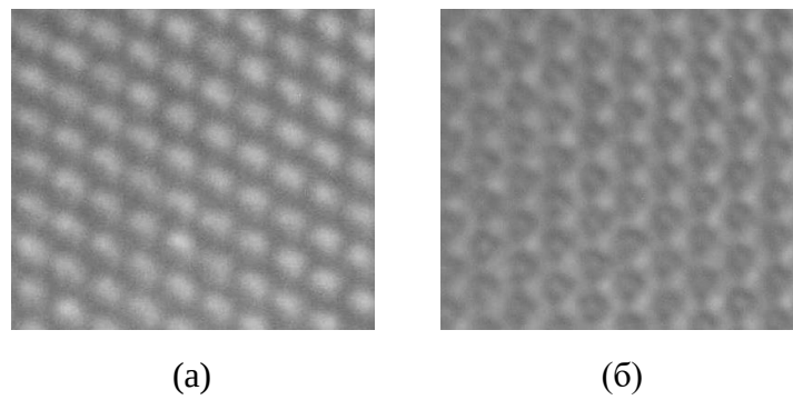
Рис. 3.12. Розподіл інтенсивності в інтерференційній картині для формування 2D фотонних кристалів при: 1) \Psi_{3,0} (а) і \Psi_{6,3} (б); 2) \Psi_{4,0} (в) і \Psi_{4,1} (г). [103]
