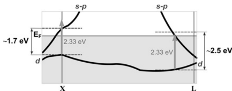
Рис. 4.2. Діаграма енергетичних рівнів, що пояснює механізм оптичної нелінійності нанокompозиту з НЧ Au [148,149].
