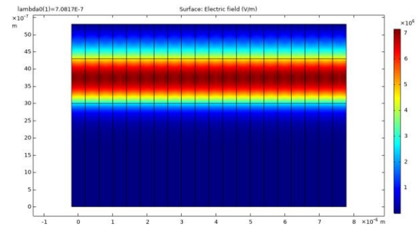
Рис. 5.8. Розподіл поля у структурі при n_s = 1,45 . Поле в підкладці є меншим (нижче ґратки), ніж у досліджуваному середовищі (вище ґратки)
