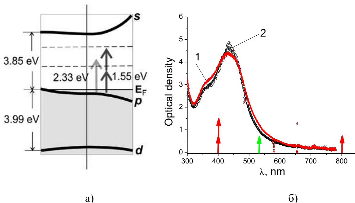
Рис. 4.6. а) Діаграма енергетичних рівнів, яка пояснює механізм оптичної нелінійності нанокompозиту Ag. б) Спектр оптичної густини полімерного нанокompозиту із вмістом НЧ Ag із хаотичною (1) і впорядкованою (2) структурою. Стрілками позначені довжини хвиль збудження: зелена стрілка відповідає \lambda_{ex} = 532 нм, h\nu = 2,33 eВ; червоні стрілки відповідають \lambda_{ex} = 800 нм, h\nu = 1,55 eВ.
