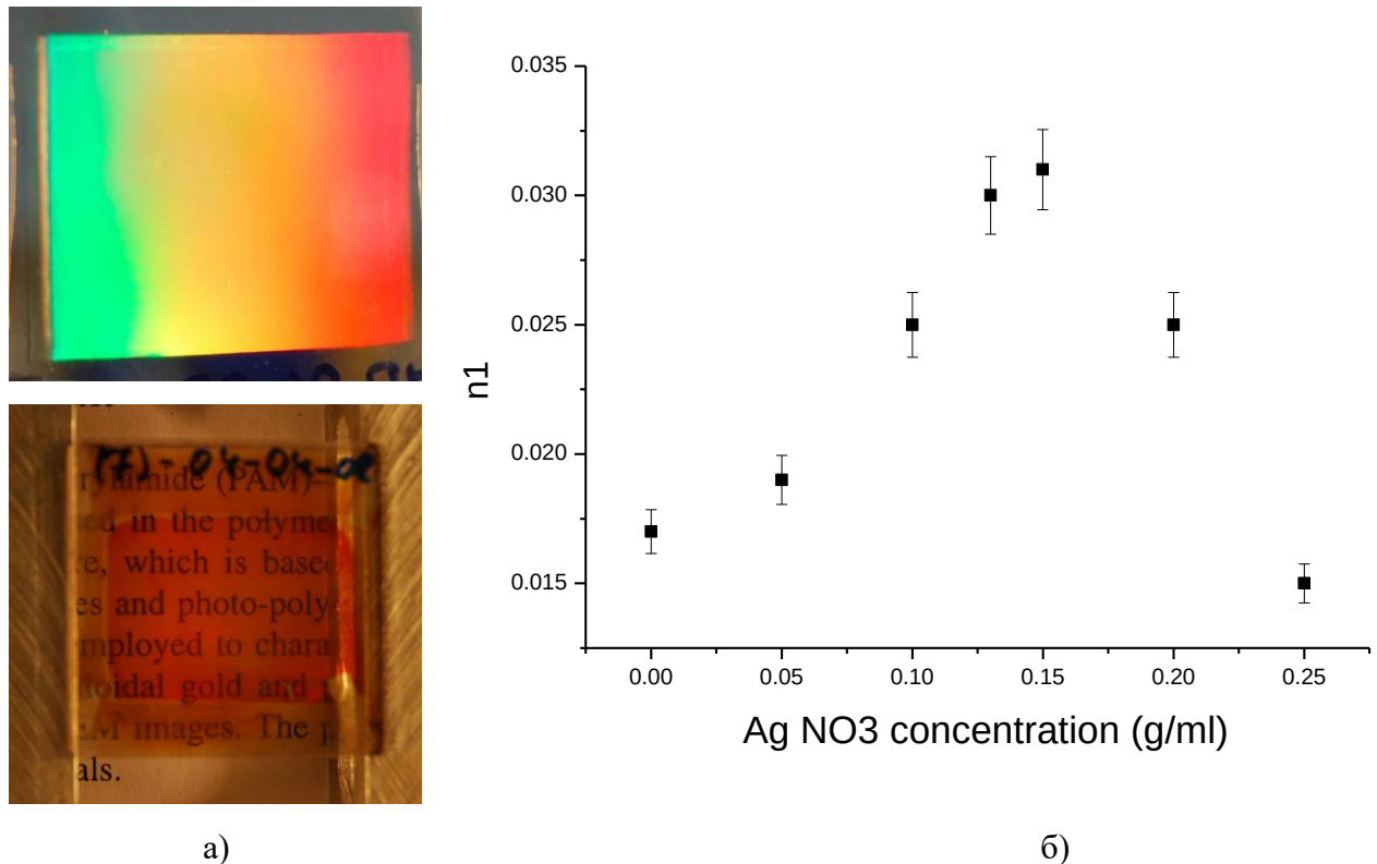
Рис. 3.9. Фото ґратки, сформованої НЧ Ag в полімерній матриці, її оптична якість (а). Залежність n_1 ґратки від концентрації \text{AgNO}_3 в розчині прекурсору (б).
