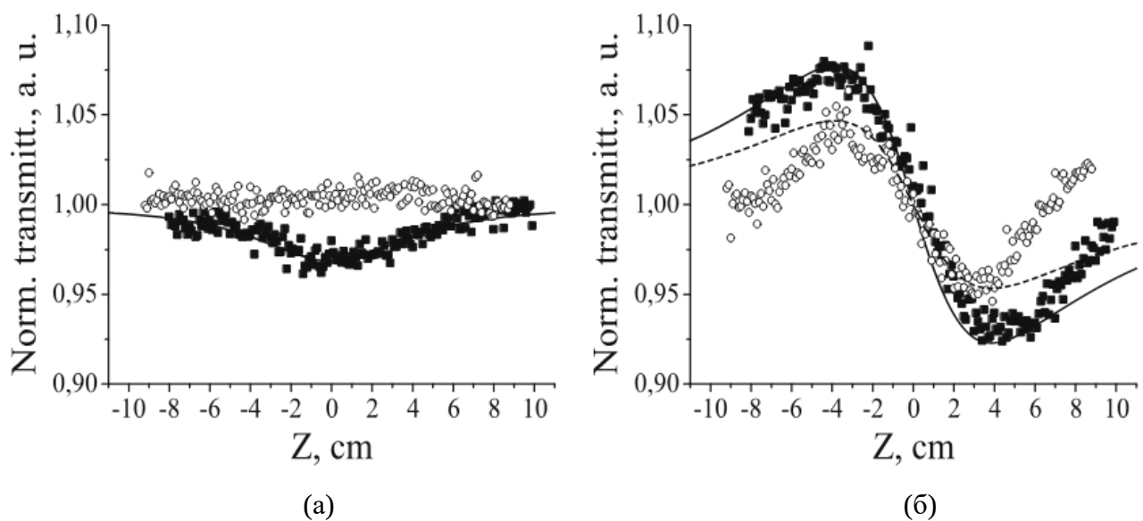
Рис. 4.5. Нелінійний відгук Ag-нанокомпозиту при збудженні на довжині хвилі 800 нм ( \tau = 180 фс, f = 75 кГц, I_0 = 0,142 ГВт/см 2 ): із відкритою діафрагмою (а) та із закритою діафрагмою (СА/ОА) (б) Результати Z-сканування для хаотичних (незафарбовані кола) і впорядкованих (чорні квадрати) структур. Лінії відповідають теоретичному наближенню.
