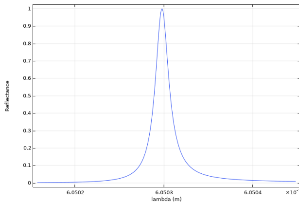
Рис.5.9. Спектральна залежність коефіцієнта відбиття при нульовому падінні світлового пучка на ґратку. Півширина спектра складає 0,0018 нм.
