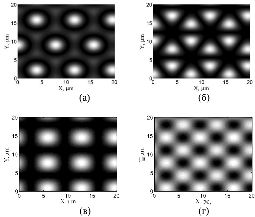
Рис. 3.12. Розподіл інтенсивності в інтерференційній картині для формування 2D фотонних кристалів при: 1) \Psi_{3,0} (а) і \Psi_{6,3} (б); 2) \Psi_{4,0} (в) і \Psi_{4,1} (г). [103]
