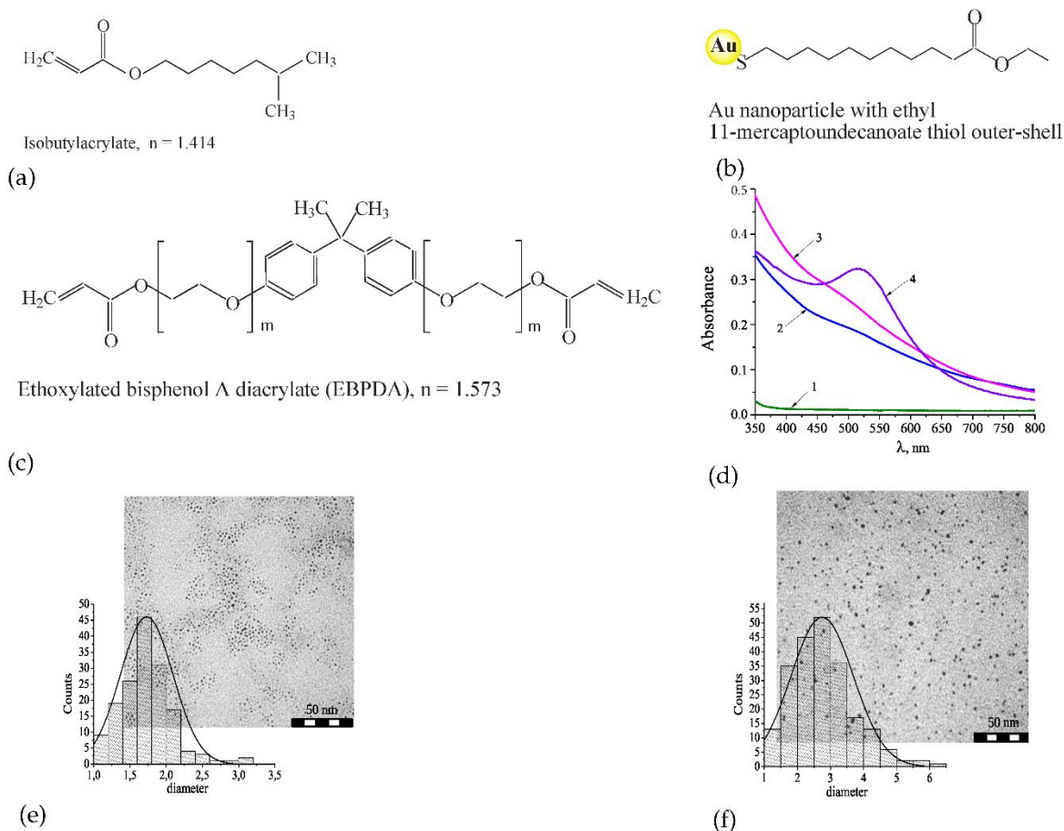
Рис. 3.3. Структурні формули компонентів композиту (а-с). Оптичні спектри шарів без та із НЧ Au (d). Мікрофотографії TEM і гістограми розподілу НЧ Au (e-f). [102]
