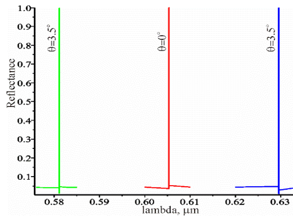
Рис. 5.3. Спектральні залежності коефіцієнта відбиття при нормальному падінні плоскої хвилі (червона крива) та при куті падіння на хвильовод 3,5^\circ (зелена та синя крива).
