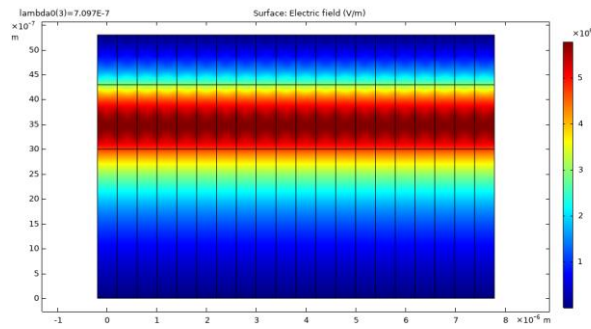
Рис. 5.7. Розподіл поля у структурі при n_s = 1,515 . Поле в підкладці є більшим (нижче ґратки), ніж у досліджуваному середовищі (вище ґратки)
