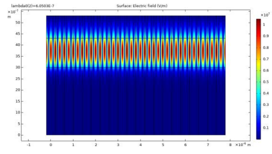
Рис. 5.6. Розподіл поля у структурі при n_s = 1,45 . Поле в підкладці є меншим (нижче ґратки), ніж у досліджуваному середовищі (вище ґратки)
