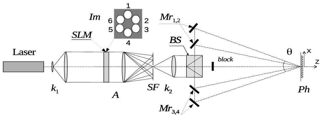
Рис. 3.11. Схема багатопучкового голографічного запису 2D структур: Laser — Ar+ лазер, k_1, k_2 — коліматори, SLM — просторовий модулятор світла, із заданим просторовим розподілом фаз Im , SF — просторовий фільтр, BS — призмове розділення лазерного пучка, Mr_{1-6} — дзеркала, \theta — кут між пучками та віссю Z, Ph — фоточутливе середовище [106,103]
