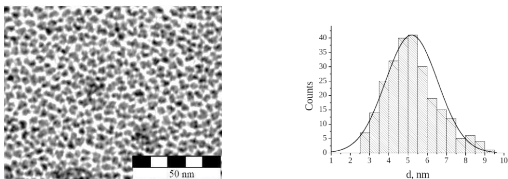
Рис. 3.2. Електронно-мікроскопічне (ТЕМ) зображення НЧ і гістограма розподілу НЧ за розміром (площа ділянки спостереження 3,5 мкм × 3,5 мкм, середній діаметр 5,24 нм, стандартне відхилення 1,37 нм).
