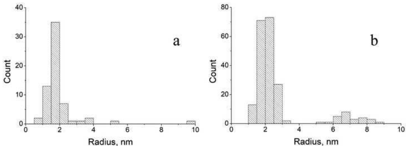
Рис. 3.17. Гістограми розподілу розмірів НЧ Ag за інтенсивності полімеризуючого випромінювання I = 14 \text{ мВт/см}^2 . (а) – У полімерному шарі (площа 1300 \text{ нм} \times 660 \text{ нм} ; середній радіус 1,7 нм; стандартне відхилення 0,3 нм). (б) – Поблизу підкладок (площа 1250 \text{ нм} \times 250 \text{ нм} ; середні радіуси 2,1 нм та 6,8 нм; стандартні відхилення 0,4 нм та 0,9 нм відповідно).
