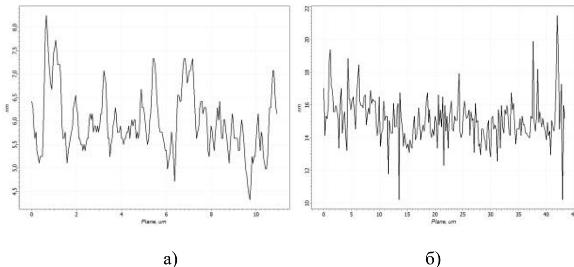
Рис. 5.13. Профілі поверхні полімерної плівки, полімеризованої між двома скляними підкладками (значення по осі Y 4,5–8,0 нм) (а) та з відкритою поверхнею на підкладці, обробленій плазмою (значення по осі Y 10,0–20,0 нм) (б); зона сканування: 10 мм × 10 мм.
