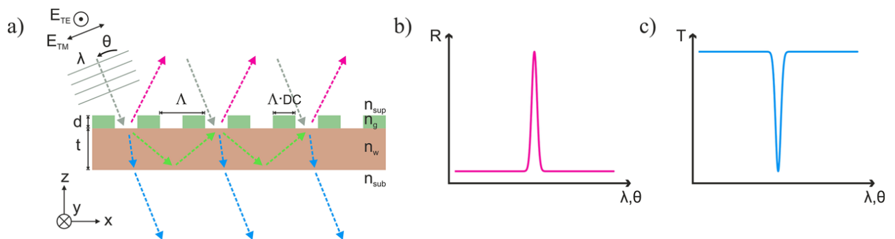
Рис. 1.1. Класична РХГ за поданням Quaranta et al. [86]. Поширення світлових променів у РХГ (а). Приклад спектрів відбиття (b) та спектрів пропускання (c) для поляризованого світла, що падає перпендикулярно до поверхні РХГ.
