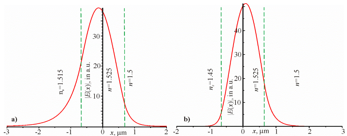
Рис. 5.4. Розподіл напруженості електричного поля у хвильоводі: а) n_s = 1,515 , б) n_s = 1,45 . Ґратка обмежена зеленими лініями. Досліджуване середовище розміщене праворуч від ґратки.
