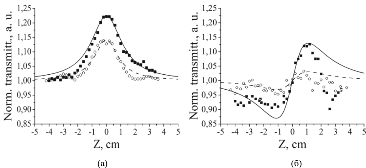
Рис. 4.4. Нелінійний відгук Ag-нанокompозиту при збудженні на довжині хвилі 532 нм ( \tau = 20 нс, f = 0,5 Гц, I_0 = 5,11 МВт/см 2 ): із відкритою діафрагмою (а) та із закритою діафрагмою (СА/ОА) (б). Результати Z-сканування для хаотичних (незафарбовані кола) і впорядкованих (чорні квадрати) структур. Лінії відповідають теоретичному наближенню.
