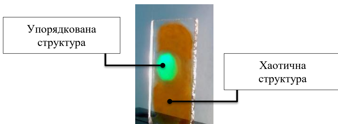
Рис. 4.3. Фотографія зразка з хаотичним і впорядкованим розподілом НЧ Ag.
