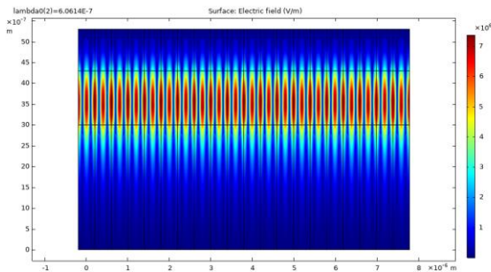
Рис. 5.5. Розподіл поля у структурі при n_s = 1,515 . Поле в підкладці є більшим (нижче ґратки), ніж у досліджуваному середовищі (вище ґратки)
