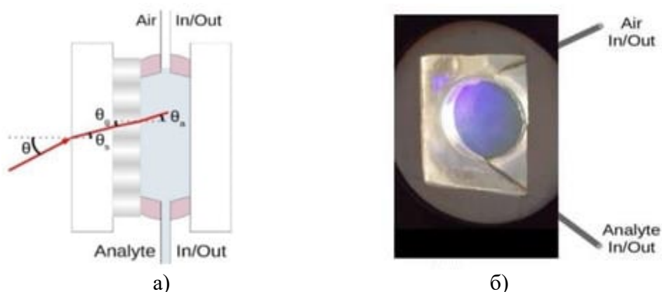
Рис. 5.16. Конструкція кювети шляхи поширення променя (а), та фото кювети (б). Стандартний метод: \theta постійний, \theta_{\text{ан}} змінюється для різних аналітів.
