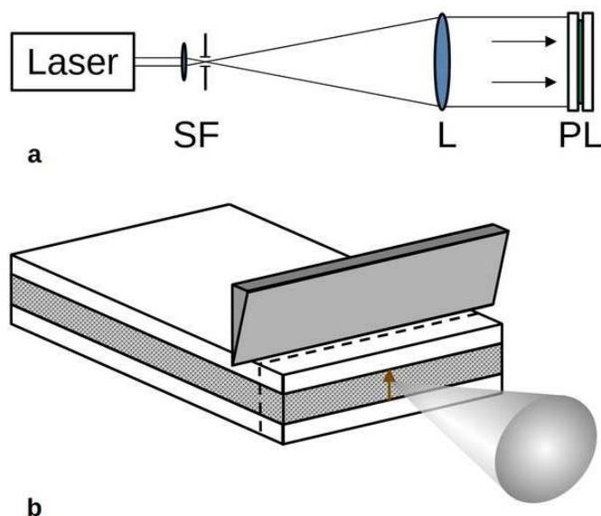
Рис.3.14. Оптична схема освітлення зразка паралельним лазерним променем: SF – просторовий фільтр, L – лінза, PL – фоточутливий шар для полімеризації. (а) Зріз зразка із використанням ультрамікротома Ultrotome III LKB 8800 для вимірювань TEM. Сканування зразка електронним променем. Напрямок сканування показано стрілкою. (b)
