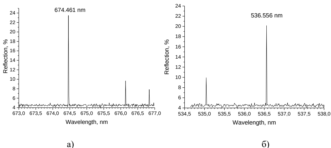
Рис. 5.15. Довгохвильові (а) і короткохвильові (б) резонансні смуги у спектрі відбиття від РХГ при падінні світлової хвилі під кутом 10^\circ .
