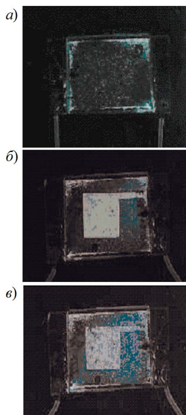
Рис. 3. Шар композита ЕББА–вуглецеві нанотрубки між схрещеними поляризаторами: а — у відсутності поля; б — в електричному полі ( U = 60 В, f = 2 кГц); в ) після вимкнення поля. Напруга прикладається до прямокутної ділянки посередині зразка.
